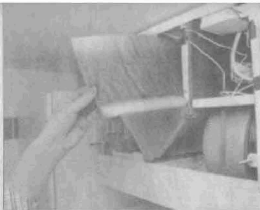
1. Katkaise laitteesta virta joko huoltokytkimestä tai irrottamalla se pistorasiasta. Avaa kansi ja irrota karkeasuodattimet.
