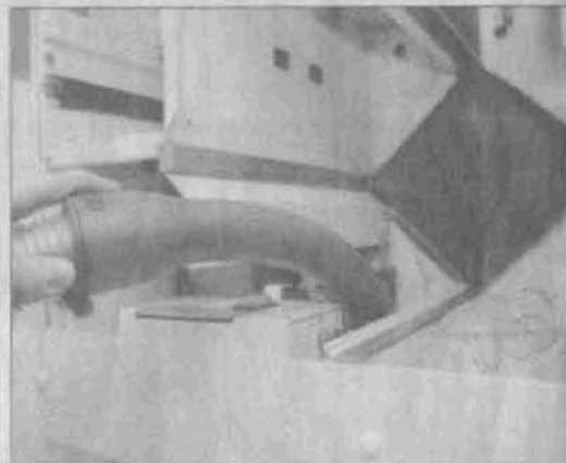
6. Imuroi ilmanvaihtolaitteen sisäosat puhtaaksi ennen kuin laitat suodattimet ja kennon takaisin.
