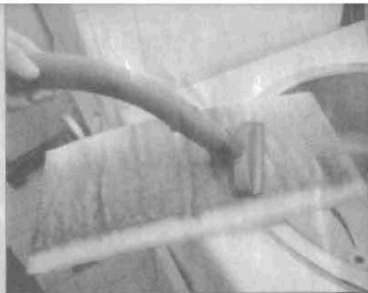
2. Imuroi suodatin tai vaihda se tarvittaessa uuteen. Se on hyvä vaihtaa uuteen syksyllä ja keväällä ja imuroida siinä välillä.
